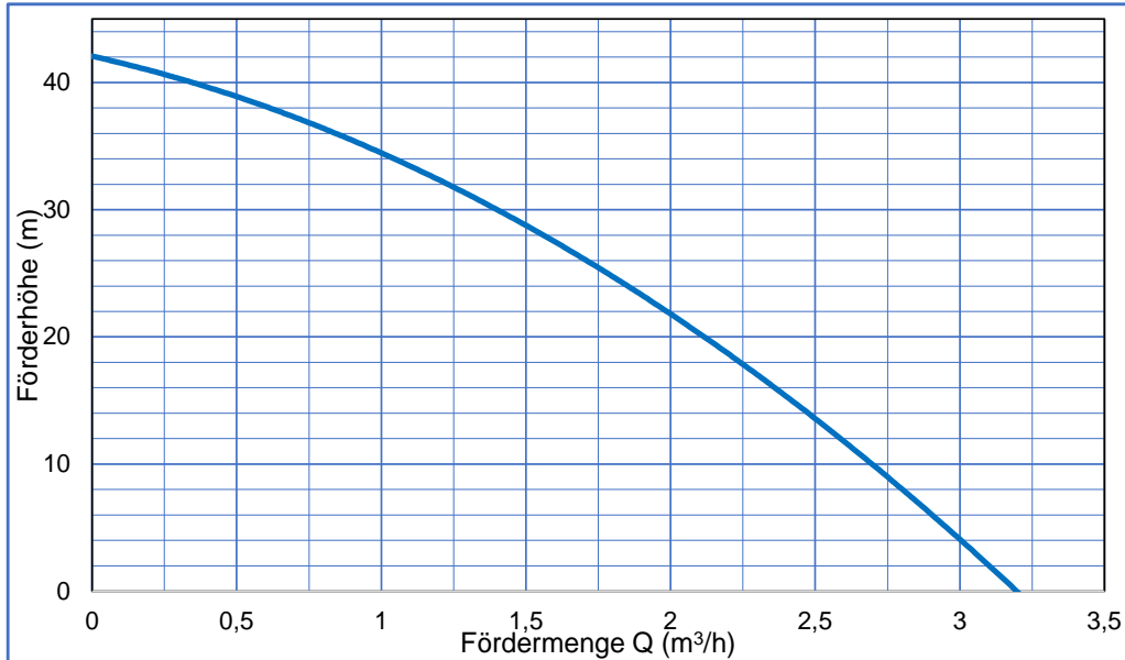
Kennlinien D-EBOOST
