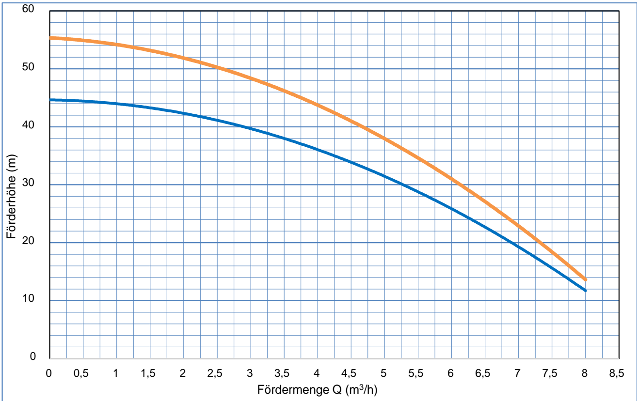
Kennliniendiagramm PowerRain plus
